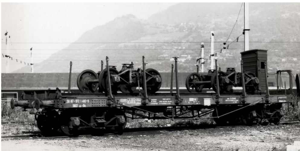
Photo : J.P. Demoy – Plat avec Guérite et Rancher et marquage UIC
