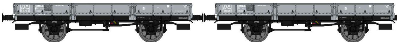
Réf. WB-600 – Set de 2 Plats OCEM 29 Gris PLM NNTouw 57789 et NNTouw 58169 Frein à levier, Roues rayons Ep.II
