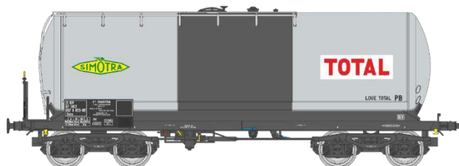
WB-589 – Citerne ANF courte bogie Y 25 Ep.IV "SIMOTRA-TOTAL"
